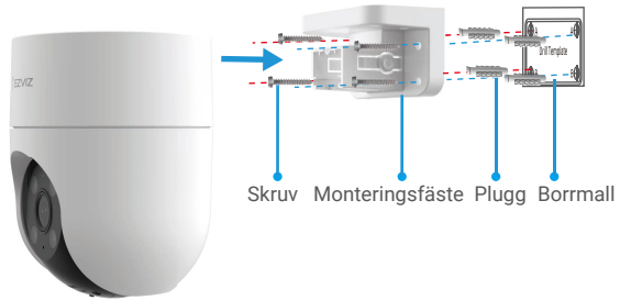
Fig. 2 Vägghmontering
